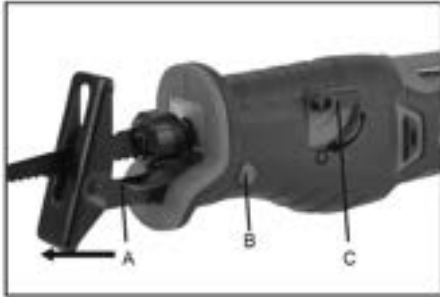
A. Shoe B. Button C. Pendulum lever
